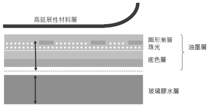
圖 2. 玻璃轉印技術結構設計圖
