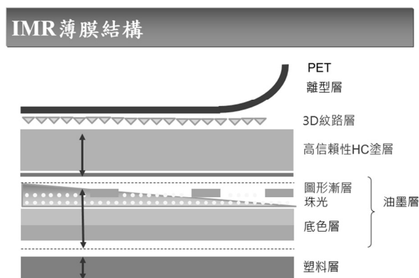
圖 1. 3D 壓紋+漸層效果薄膜之結構設計
