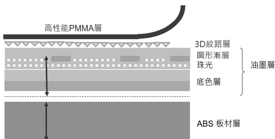
圖 6. 汽車產品的基本結構圖
