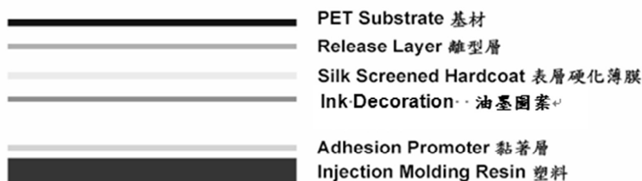
圖 1 IMR 薄膜構成圖
